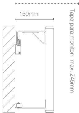
Nivel móvil con tapa para rail
